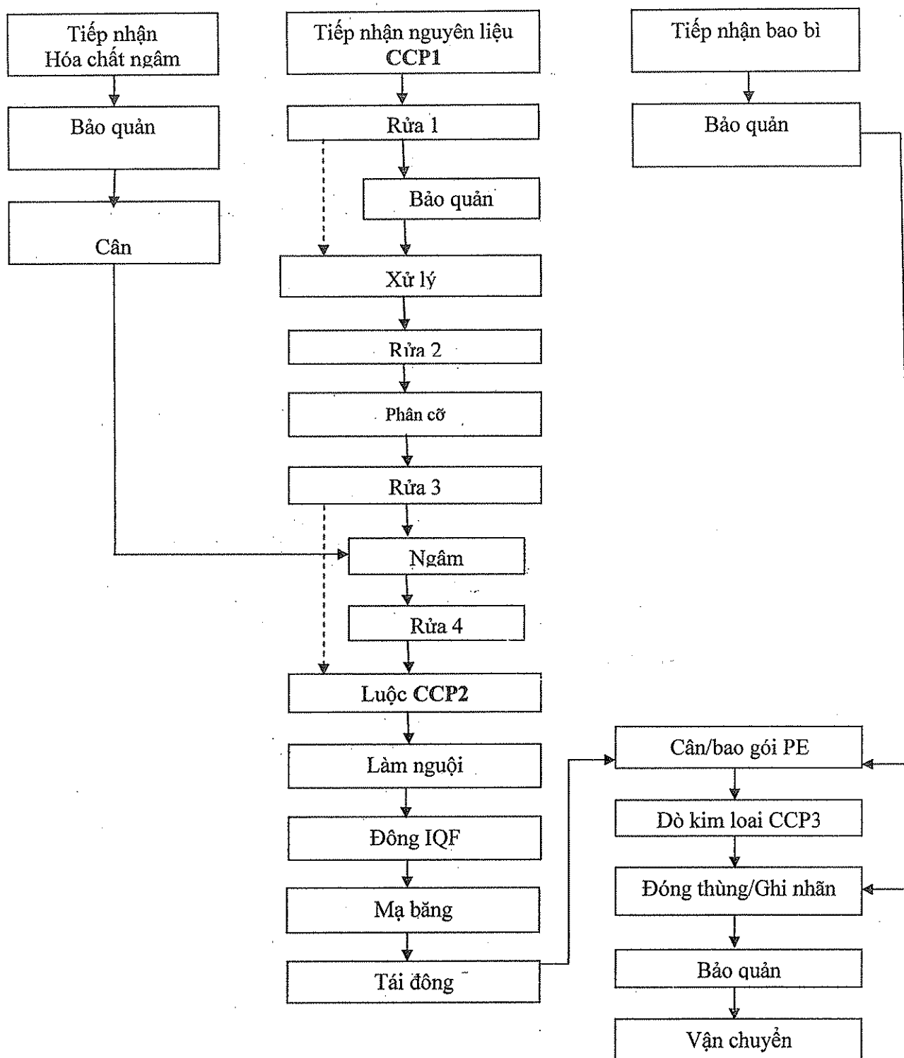
Hình 5: Quy trình công nghệ chế biến sản phẩm: Tôm sú luộc đông IQF
